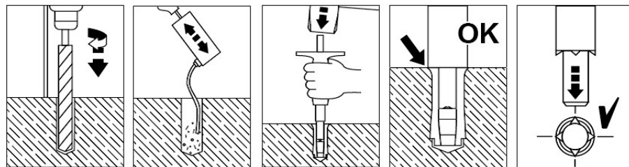
Abb. 4-2: Anleitung zum Setzen der Dübel (Quelle: Fa. Hilti)
