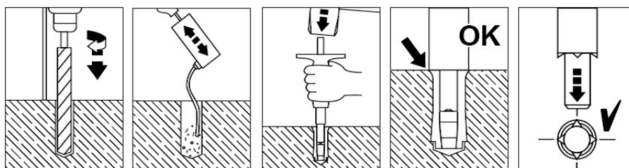
Afb. 4-2: Handleiding voor het plaatsen van pluggen (Bron: Hilti)
